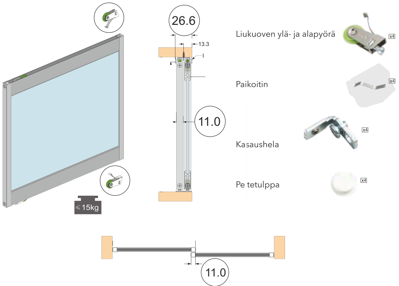
Liukuoven vaakakisko ylös ja alas
