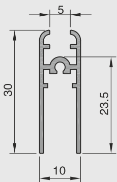
Liukuoven vaakakisko ylös ja alas
